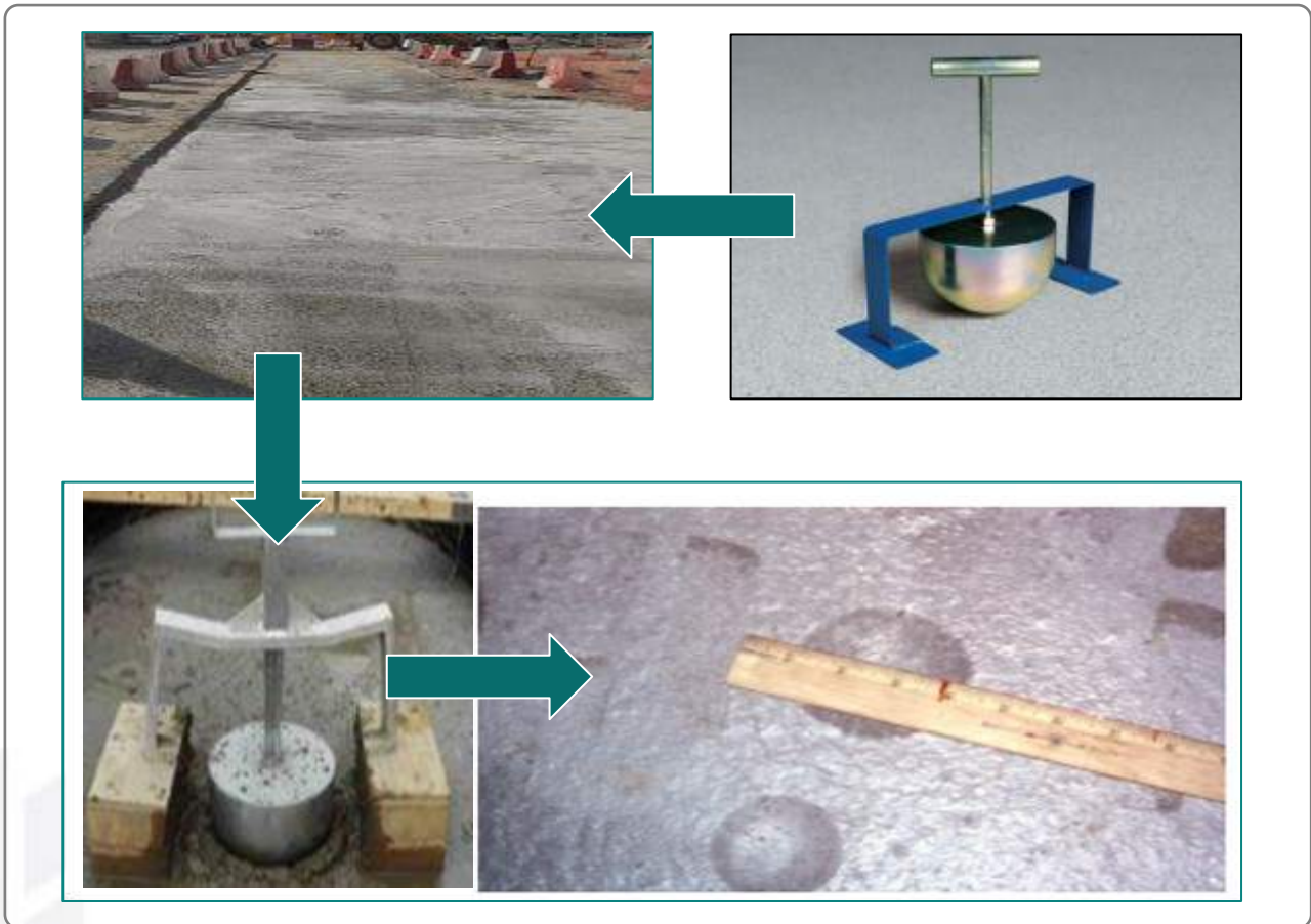
الشكل (5): اختبار مقاومة الاختراق باستخدام (كرة كيلبي) للتأكد من تصلب مواد (الخرسانة الرغوية)
