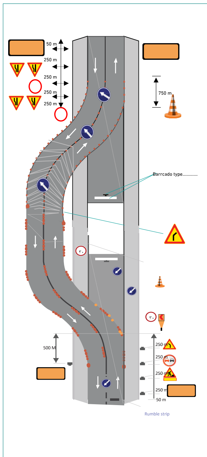
الشكل (12): منطقة عمل حارة واحدة على طريق مكون من حارتين -حالة الكتف المرصود
