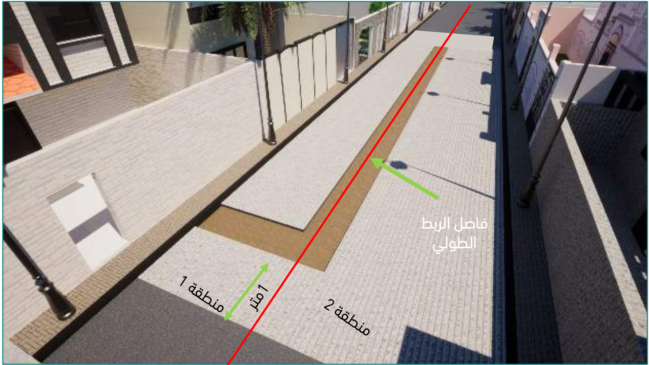
الحفرة حال وقوعها على فاصل الربط الطولي بشكل V أو ٨
