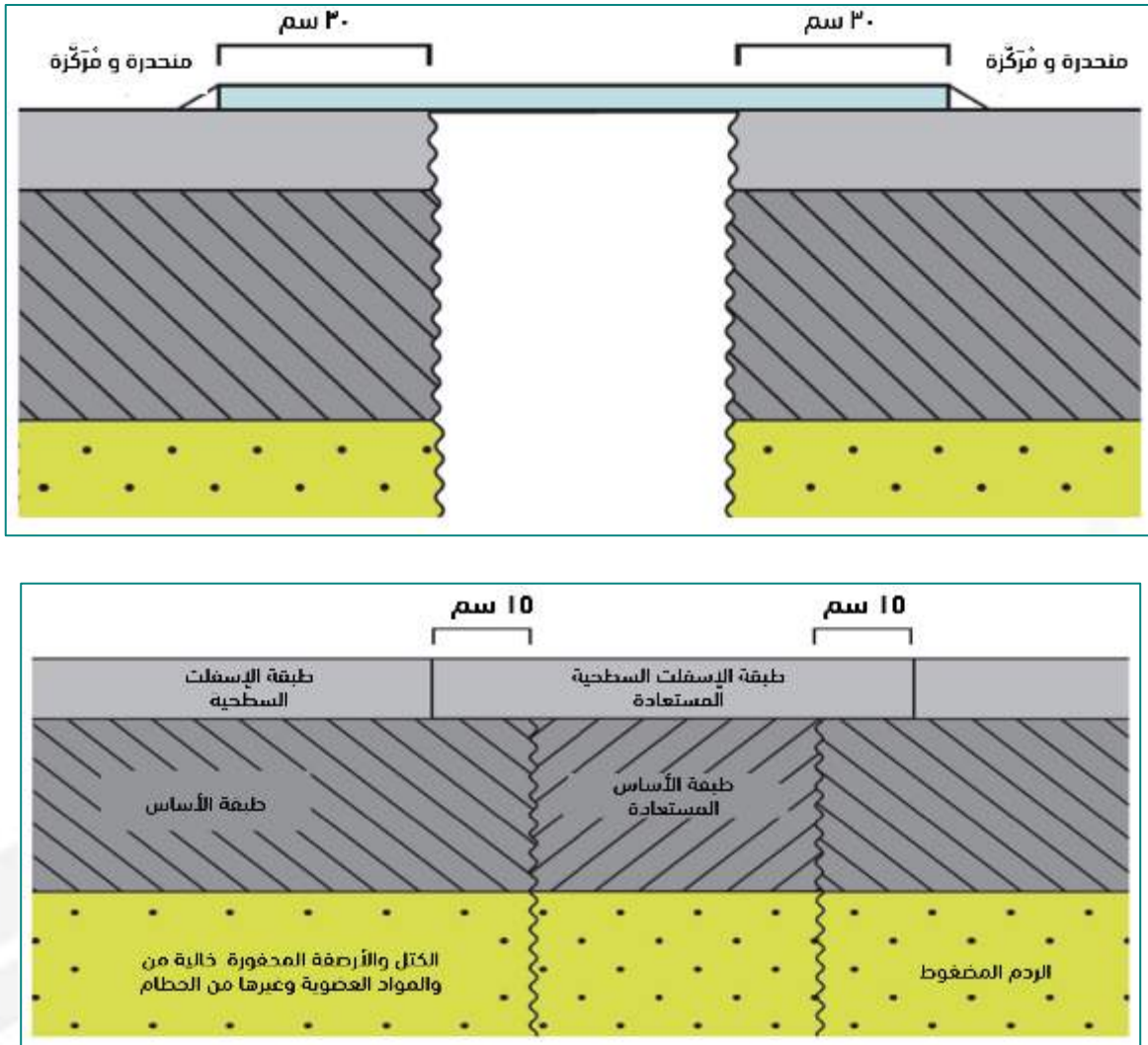
الشكل (14): إقفال مواقع الحفر في حالة إغلاق الطرق لمدة طويلة
